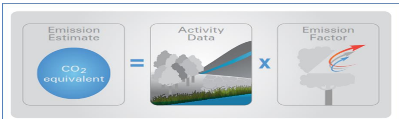
Figure 5 : Formule de calcul des émissions du GIEC
