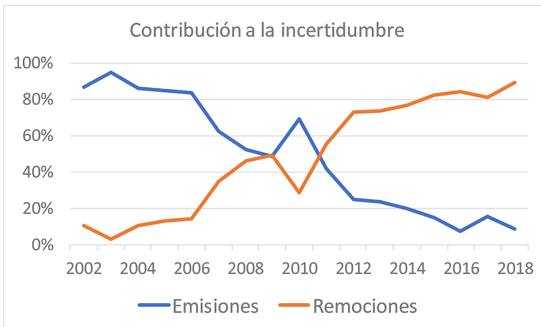
Figura 19. Tendencias en la contribución de las actividades que generan emisiones y actividades que generan remociones a la incertidumbre del NRF (Disponible en Incertidumbre NRF 90CI-AnualFinal. xlsx)
