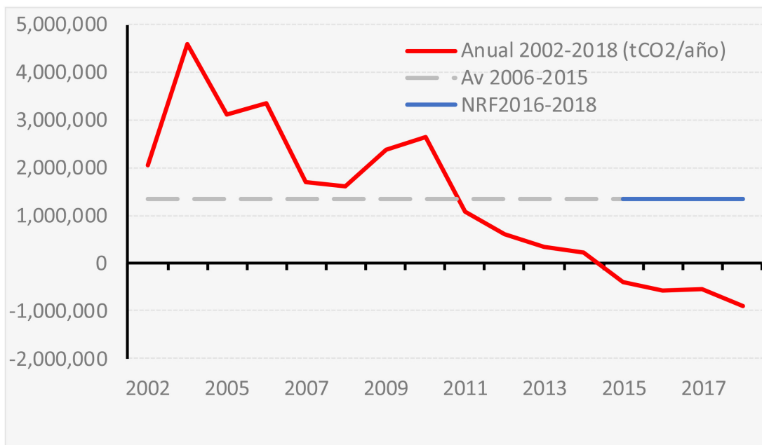
Figura 13. Tendencia en el total de emisiones/remociones anuales (en tCO 2 /año) entre 2001–2018, promedio de emisiones del periodo histórico de 2006–2015 y diferencia entre NRF2016–2018 y emisiones anuales 2016–2018.
