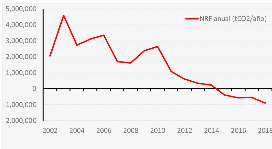
Figura 12. Tendencia en el total de emisiones/remociones anuales (en tCO 2 /año) entre 2001-2018 para El Salvador, incluyendo emisiones de COS por deforestación y remociones de COS por reforestación.
