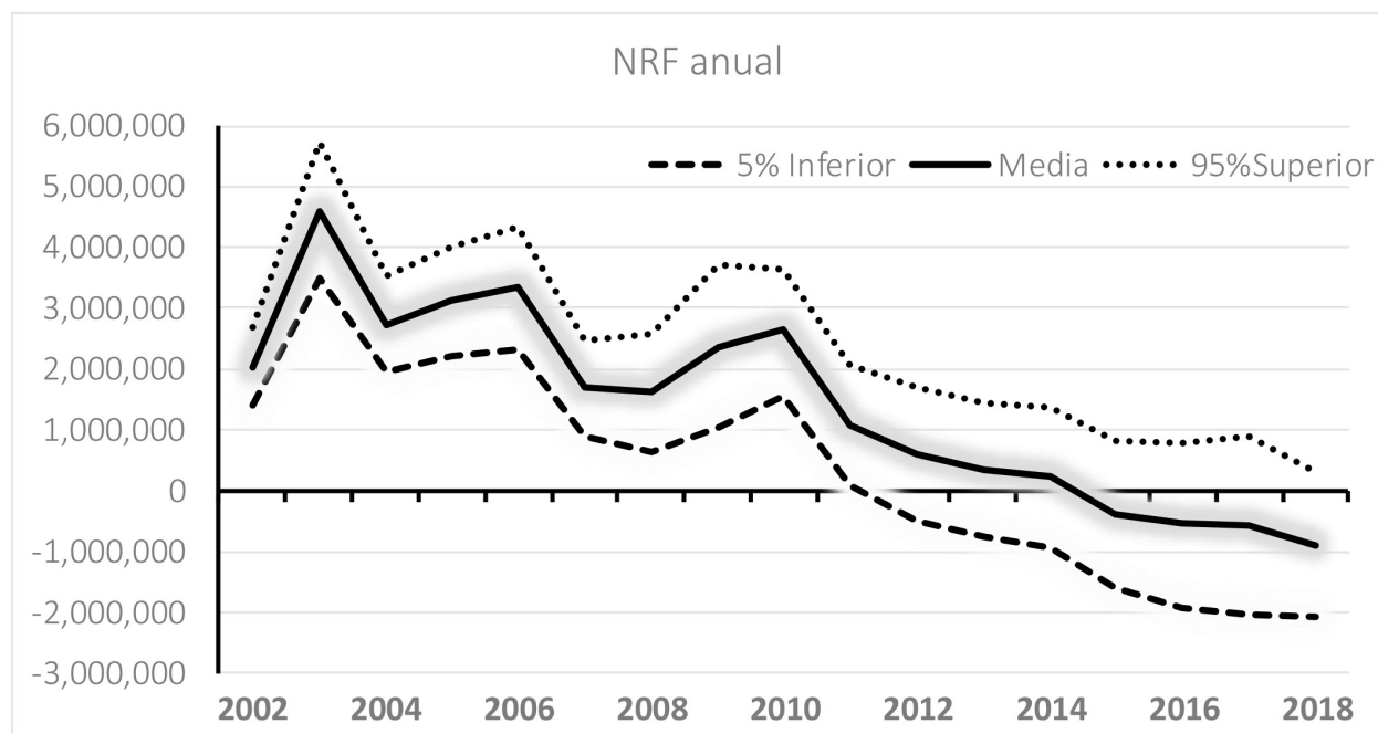
Figura 18. Tendencia en las emisiones anuales con los niveles de 5 % inferior y 95 % superior de la distribución de los resultados de las 5,000 simulaciones (Disponible en Incertidumbre NRF 90CI-AnualFinal.xlsm).
