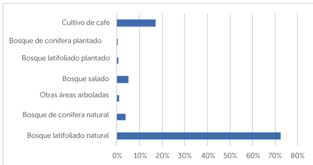
Figura 3. Proporción de cobertura forestal en 2011
